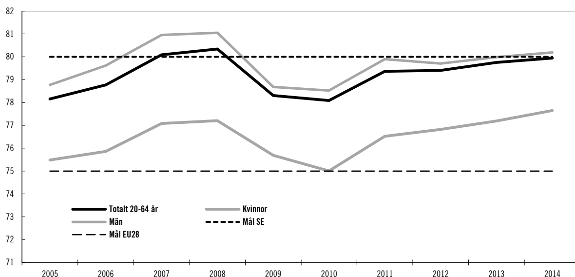
Diagram 1. Utvecklingen av sysselsättningen för åldersgruppen 20–64 år 2005–2014 kontrasterad mot Europa 2020 målet för Sverige (väl över 80 %) samt för hela EU (75 %)
