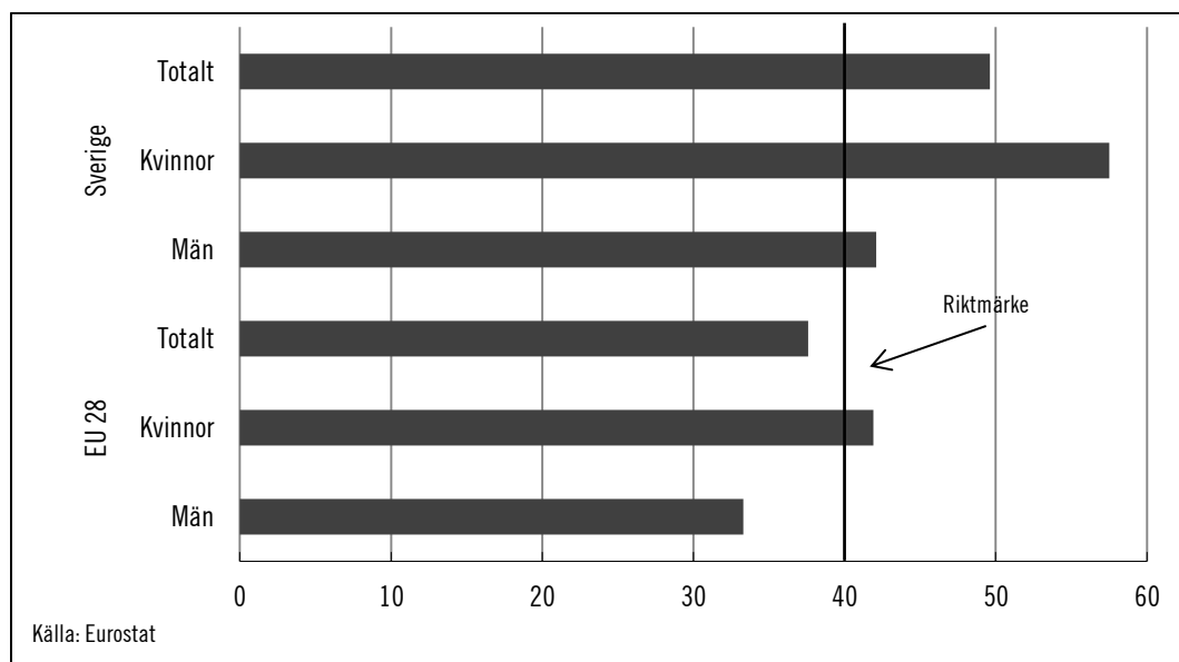
Diagram 2: Andel i åldern 30–34 år med minst två års eftergymnasial utbildning (2014)
